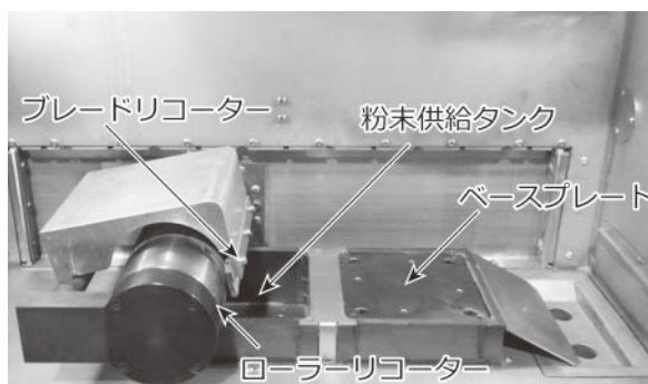
図2 金属3Dプリンターの装置内部
