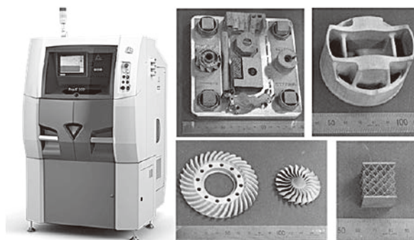
図1 金属3Dプリンターの外観と造形事例
